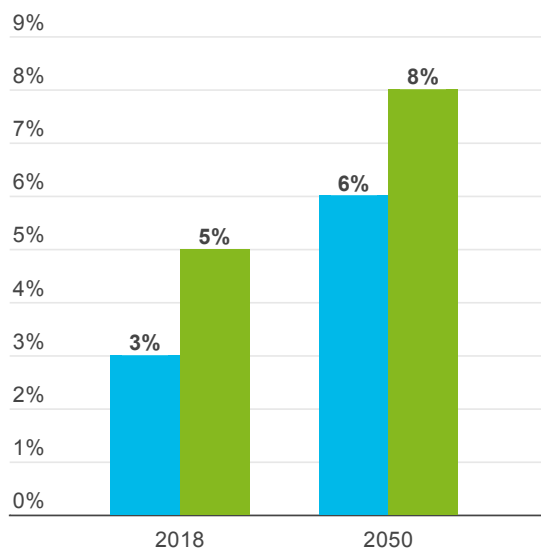
Grafiek 15 | Evolutie gebouwen met wateroverlast ten gevolge van intense neerslag, t.o.v. gebouwen (huidige klimaat en 2050)
