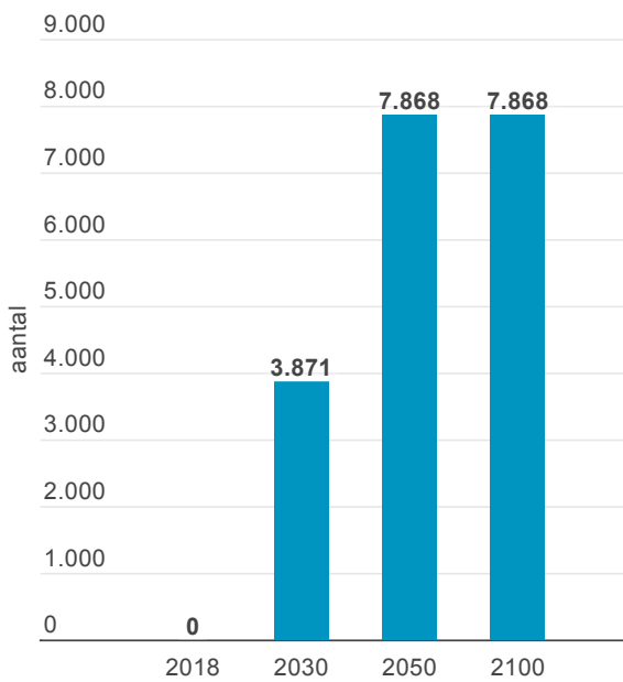
Grafiek 19 | Evolutie door hitte getroffen kwetsbare inwoners (0-4 jaar en 65+ jaar) in Asse (huidige klimaat, 2030, 2050 en 2100)
