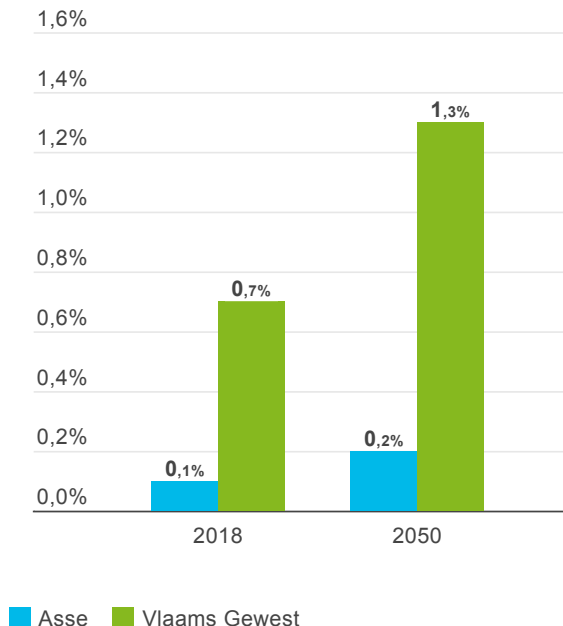
Grafiek 13 | Evolutie overstroombare gebouwen bij overstroming vanuit waterlopen, t.o.v. totaal aantal gebouwen (huidige klimaat en 2050)
