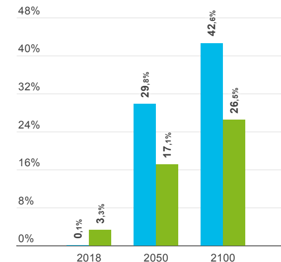
Grafiek 6 | Evolutie oppervlakte kwetsbare ecotopen met significante droogtestress, % t.o.v. oppervlakte (huidige klimaat, 2050 en 2100)
