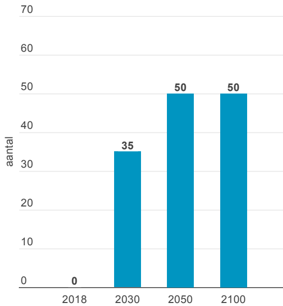
Grafiek 20 | Evolutie kwetsbare instellingen met hittestress in Asse (huidige klimaat, 2030, 2050 en 2100)
