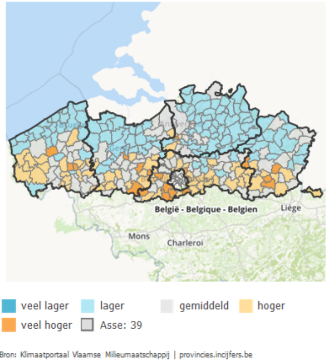
Kaart 10 | Maximale waterdiepte (2050) (z-scores)
