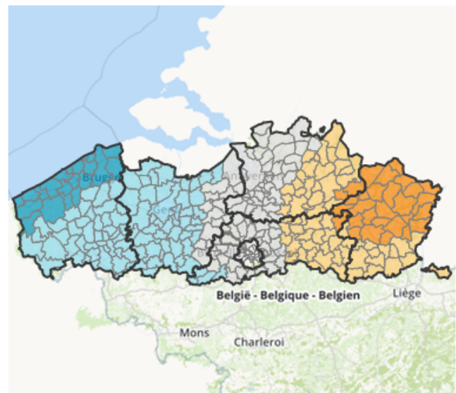
Kaart 11 | Tropische dagen per jaar (2100) (z-scores)
