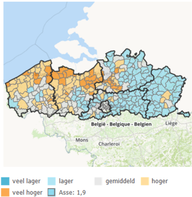
Kaart 5 | Gemiddeld laagwaterdebiet (2100) (z-scores)
