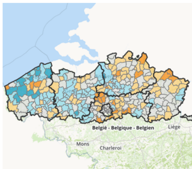
Kaart 7 | Oppervlakte kwetsbare ecotopen met significante droogtestress, % t.o.v. oppervlakte (2100) (z-scores)
