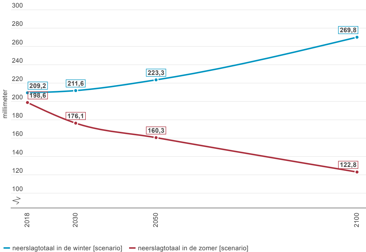
Grafiek 8 | Evolutie jaarlijkse hoeveelheid neerslag in de zomer en in de winter in mm (huidige klimaat, 2030, 2050 en 2100)
