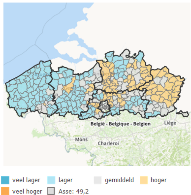
Kaart 12 | Door hitte getroffen kwetsbare inwoners 0-4 jaar en 65+ jaar, % t.o.v. 0-4 en 65+ jaar (2030) (z-scores)
