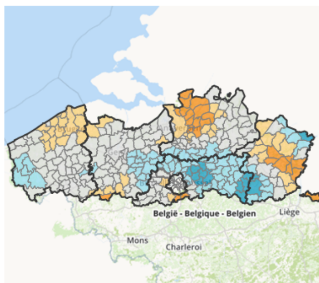
Kaart 8 | Jaarlijkse hoeveelheid neerslag (2100) (z-scores)
