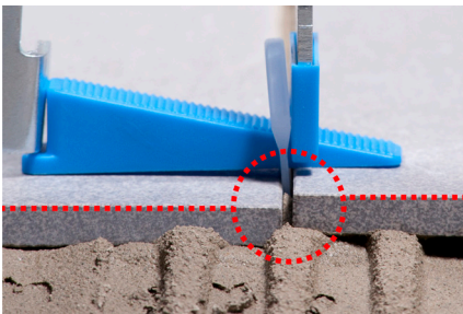
KLS nivelleersysteem
