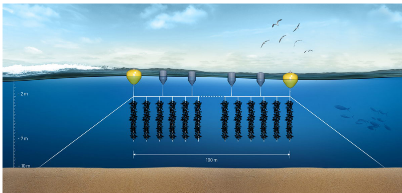
Simulatie van 1 mosselrij met 12 mosseltouwen
