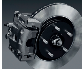
Disques de frein ventilés de 16 pouces à l'avant
