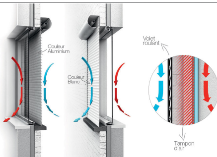
Volet extérieur VR150
