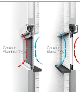
Volet monobloc OB440/OB450
